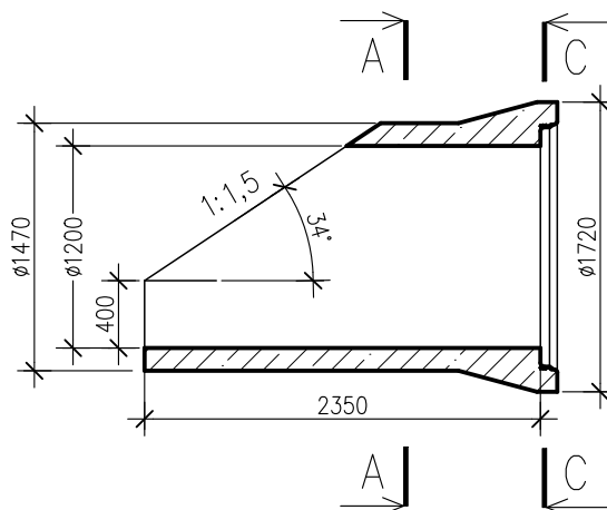
PRZEKRÓJ B-B
